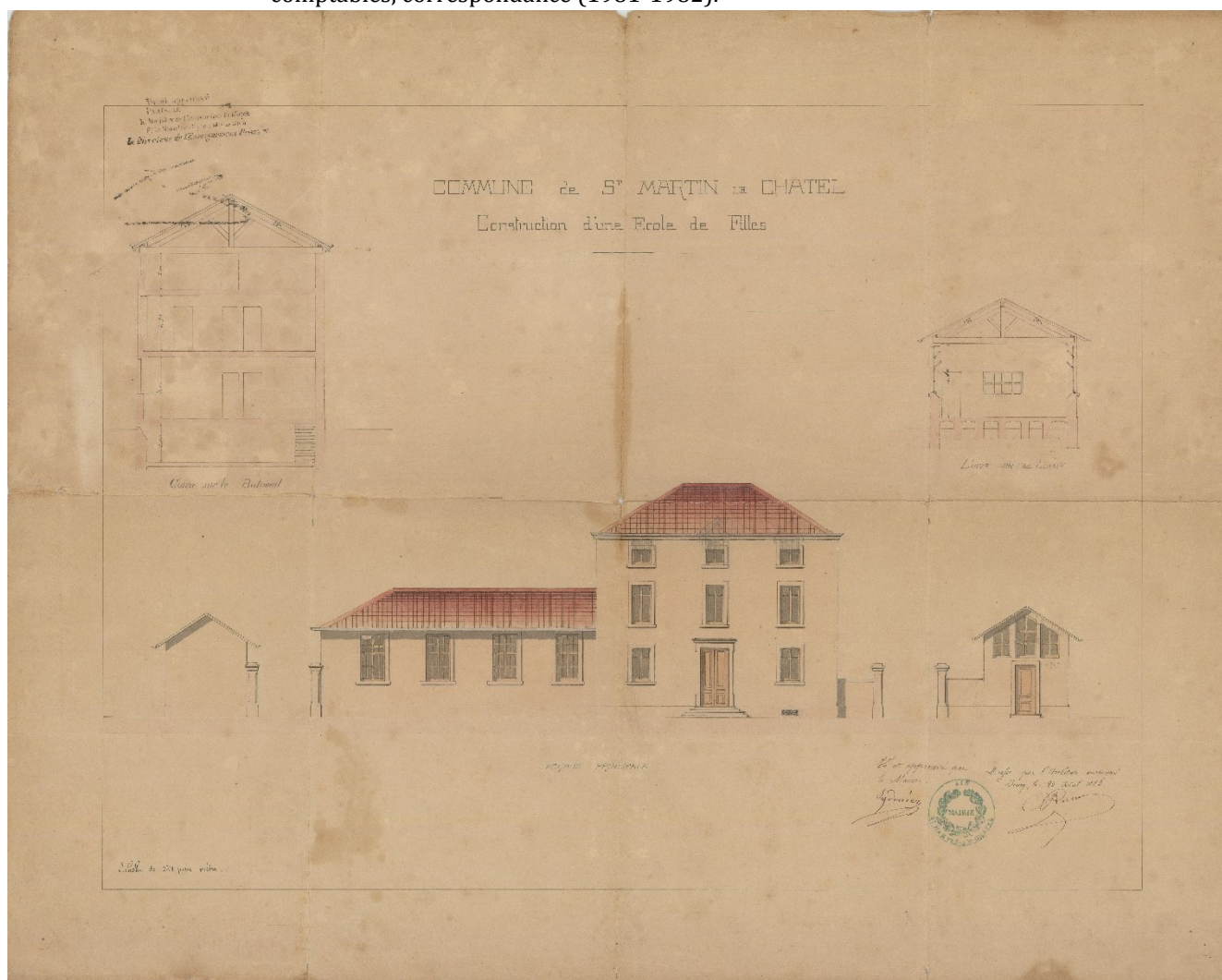
Figure 4 - Plan pour la construction d'une école de fille, 1882 (4M2).
