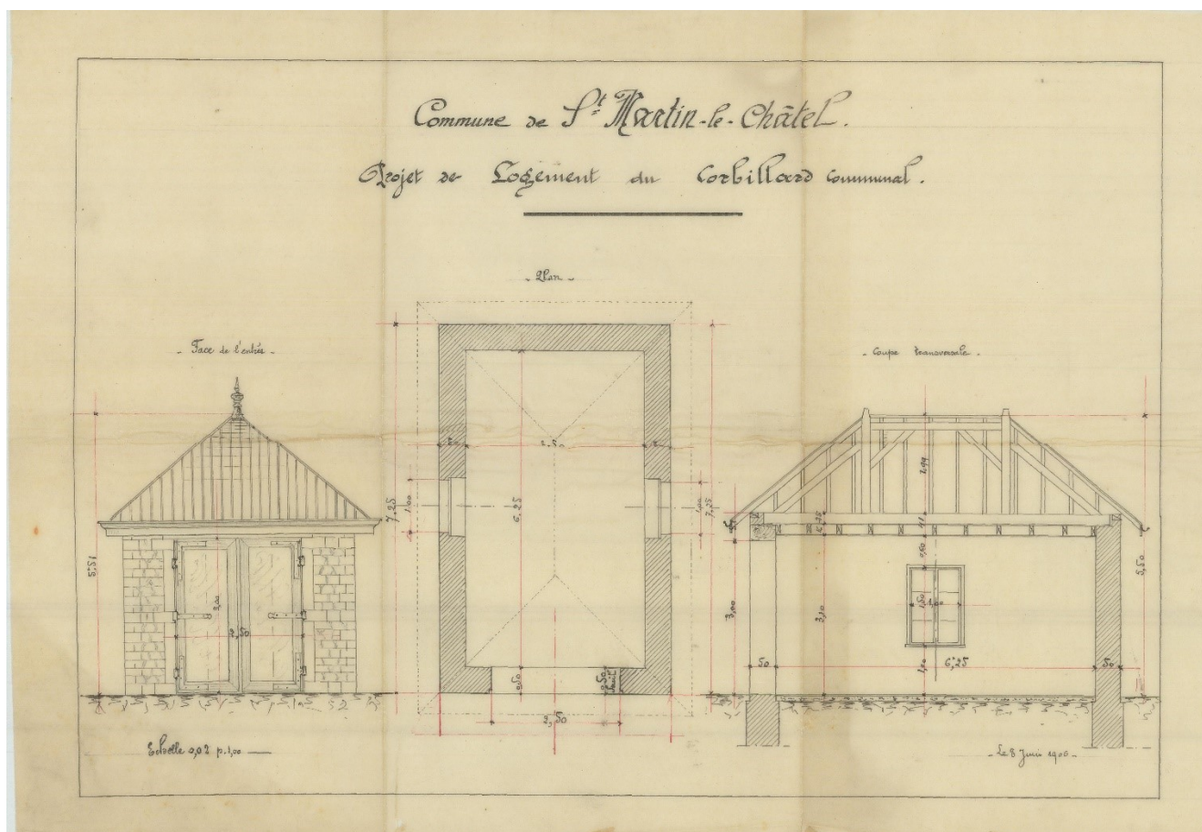
Figure 3 - Plan pour la construction d'une remise pour le corbillard, 1M3 [1906].
