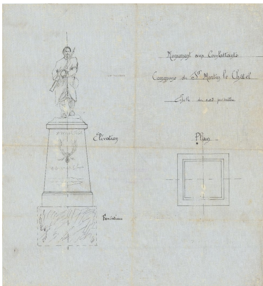
Figure 2 - Plan pour la construction du monument aux morts, 1M2 [1921].
