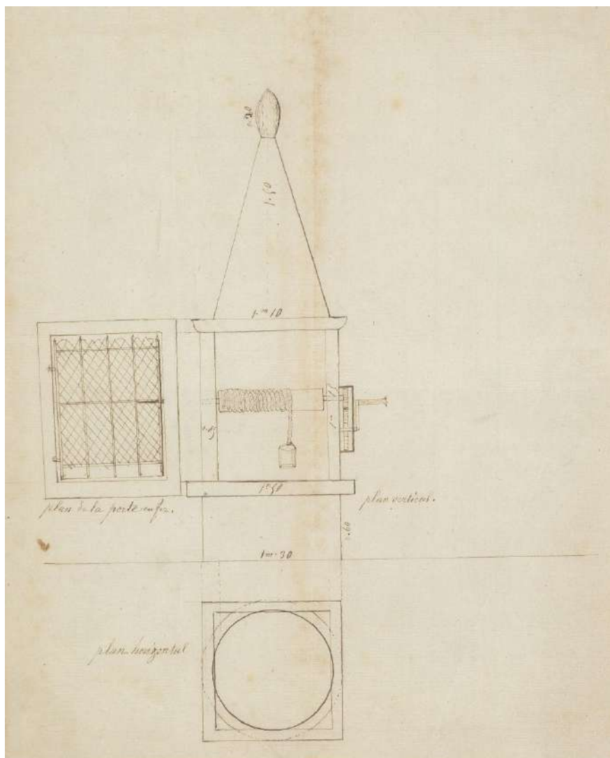
Figure 8 - Plan pour la construction d'un puits, [1858] (N2).
