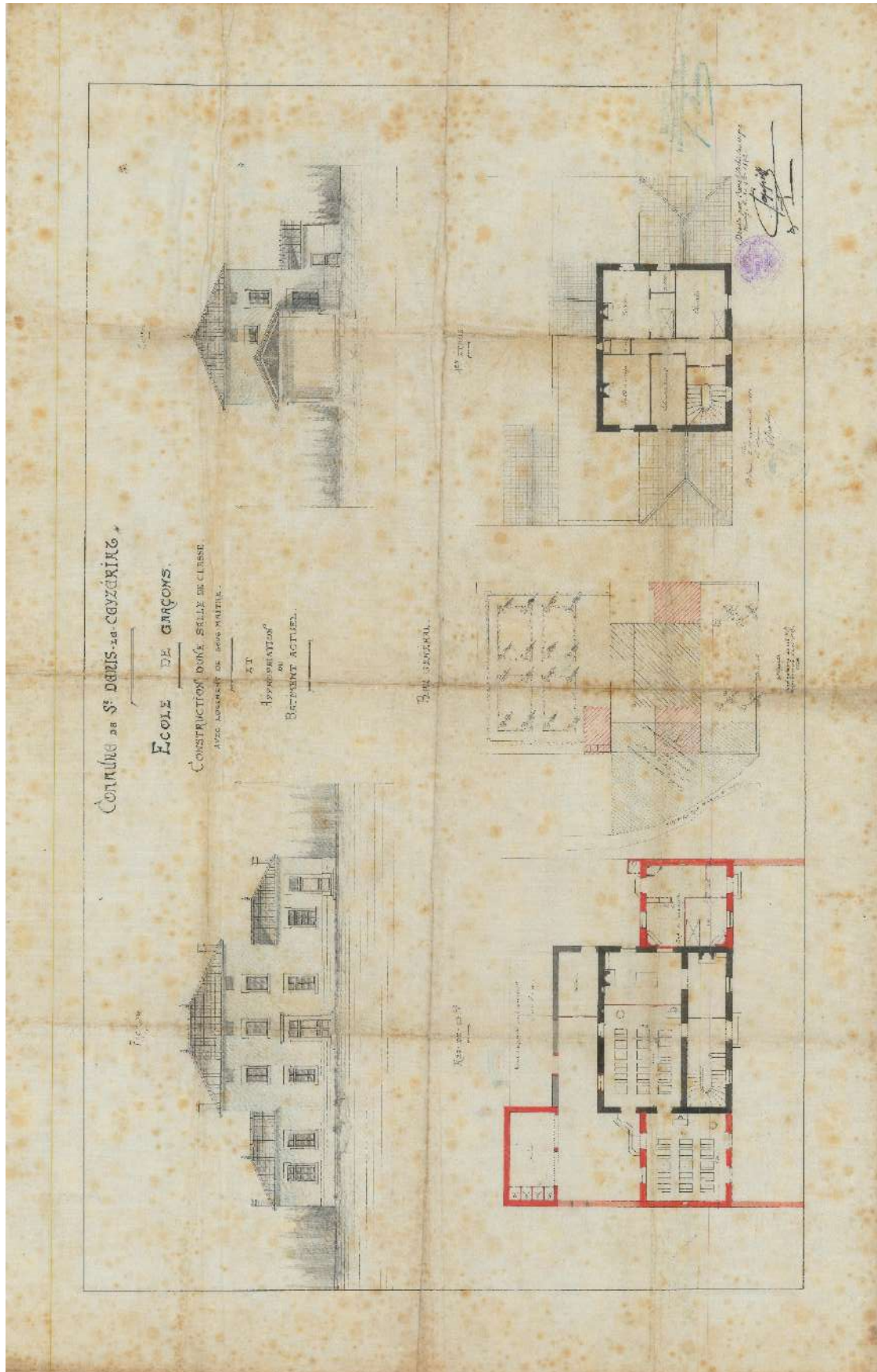
Figure 6 – Plan pour la construction d'une salle de classe avec logement de sous-maître et appropriation du bâtiment actuel à l'école des garçons, M19 (1892).
