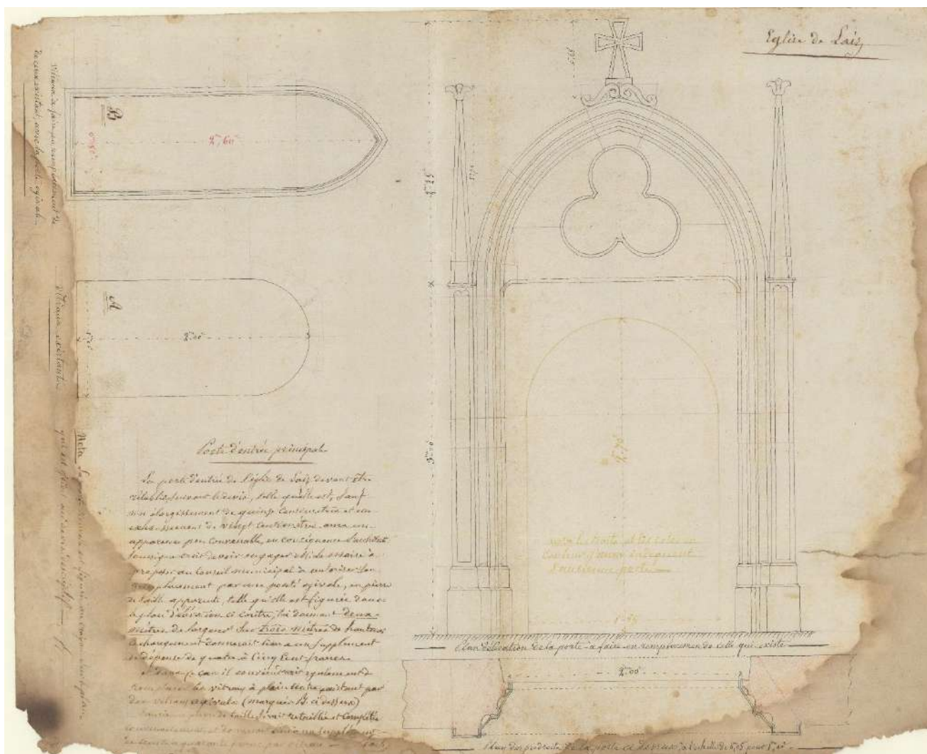
Figure 5 - Plan de la porte d'entrée principale pour l'agrandissement de l'église, milieu du 19 ème siècle (M3).
