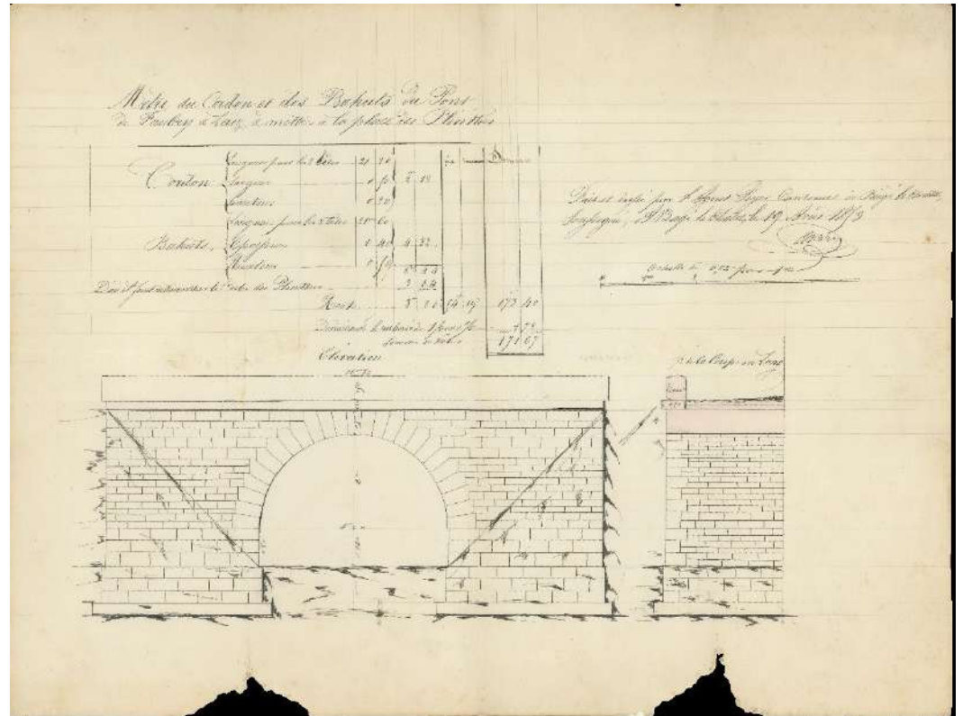
Figure 6 – Plans pour la construction d'un pont de Faubry sur le bief de Malivert, 1853 (O3).
