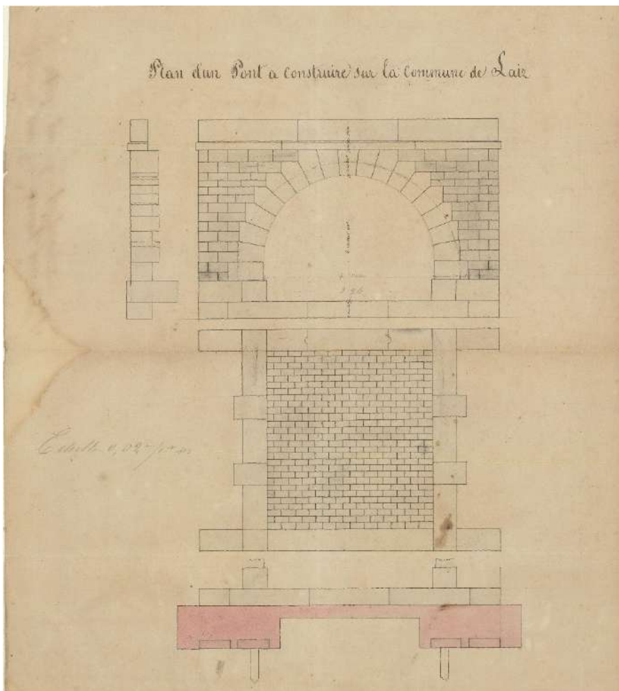
Figure 6 – Plans pour la construction d'un pont de Faubry sur le bief de Malivert, 1853 (O3).
