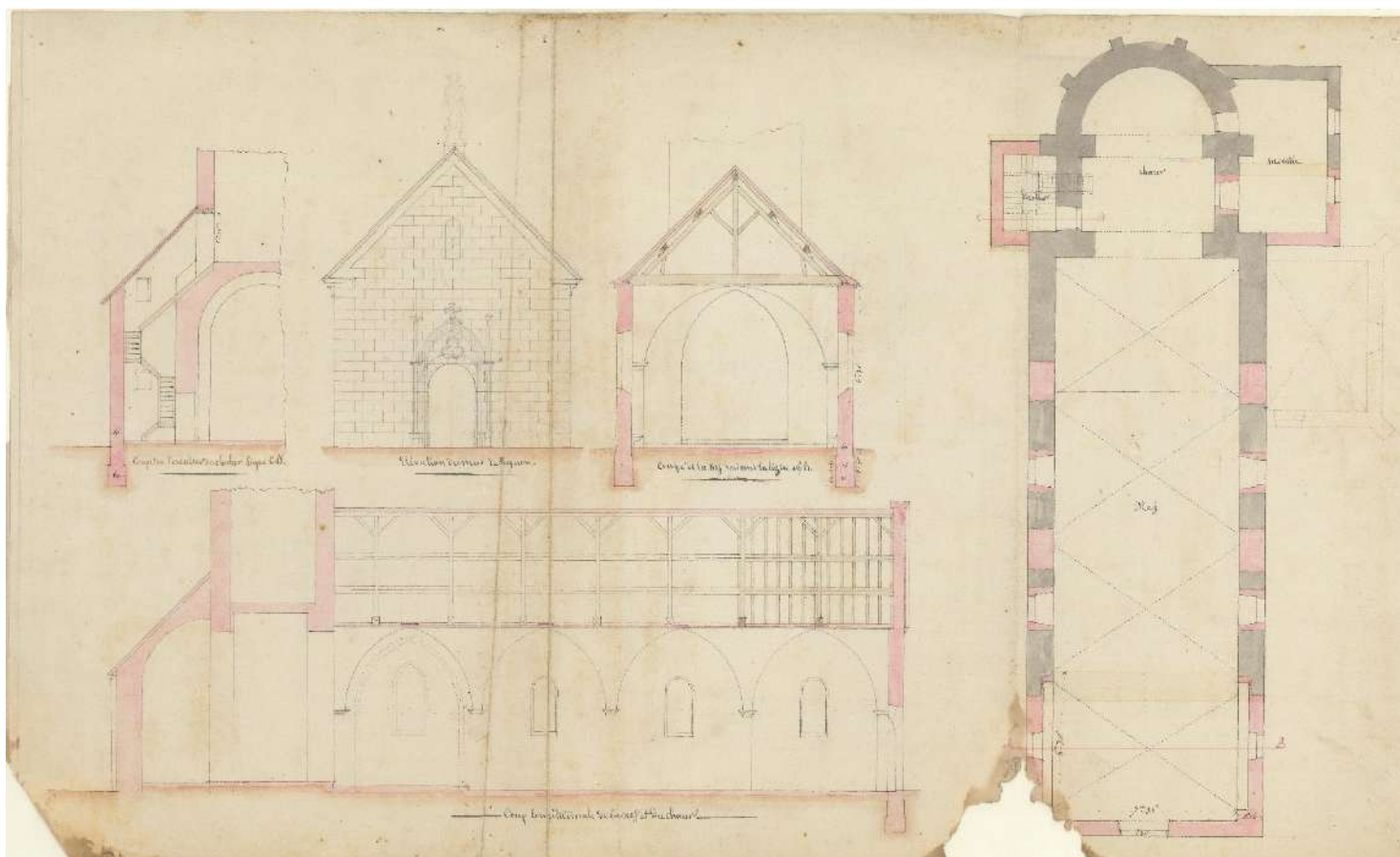
Figure 4 - Plan pour l'agrandissement de l'église, milieu du 19 ème siècle (M3).
