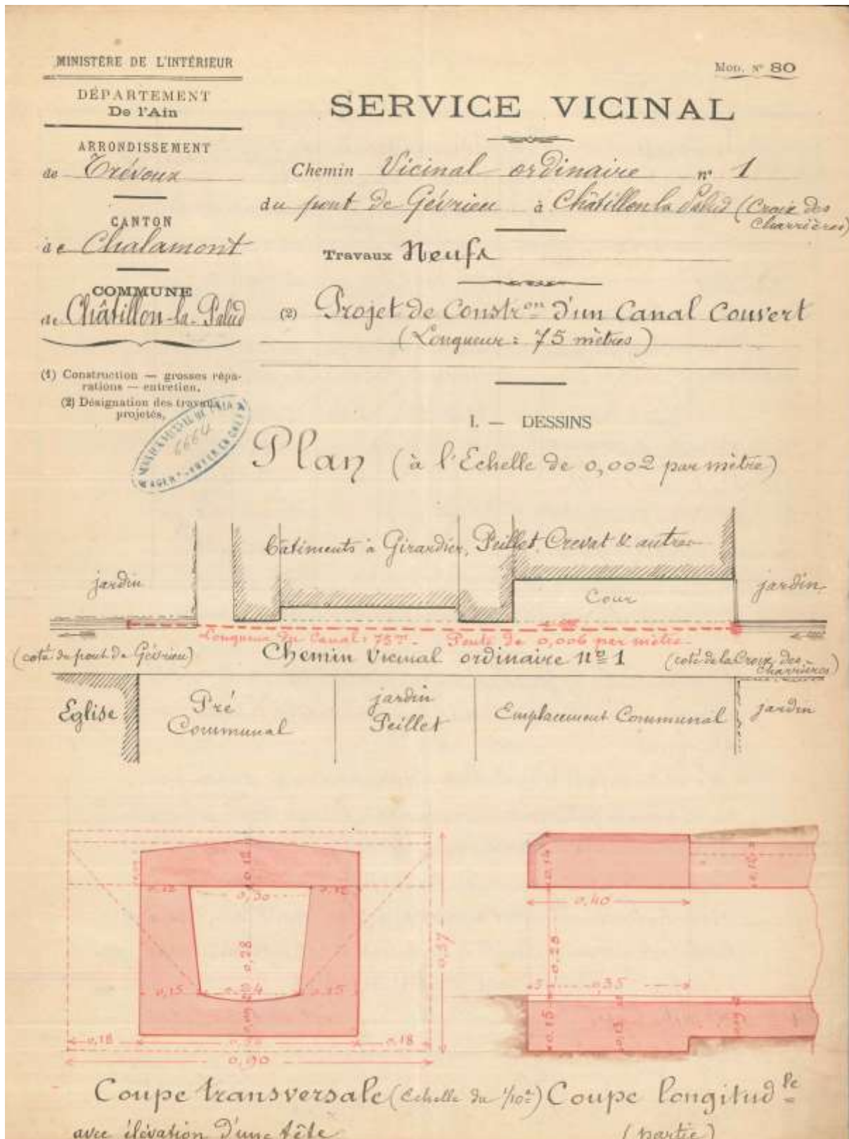
Figure 7 - Projet de canal couvert, O1 (1903)
