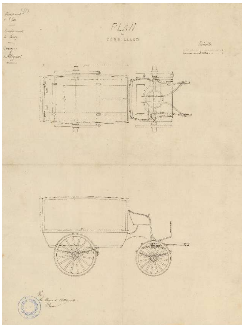
Figure 6 - Plan pour l'acquisition d'un corbillard, Fi 1 [1899].
