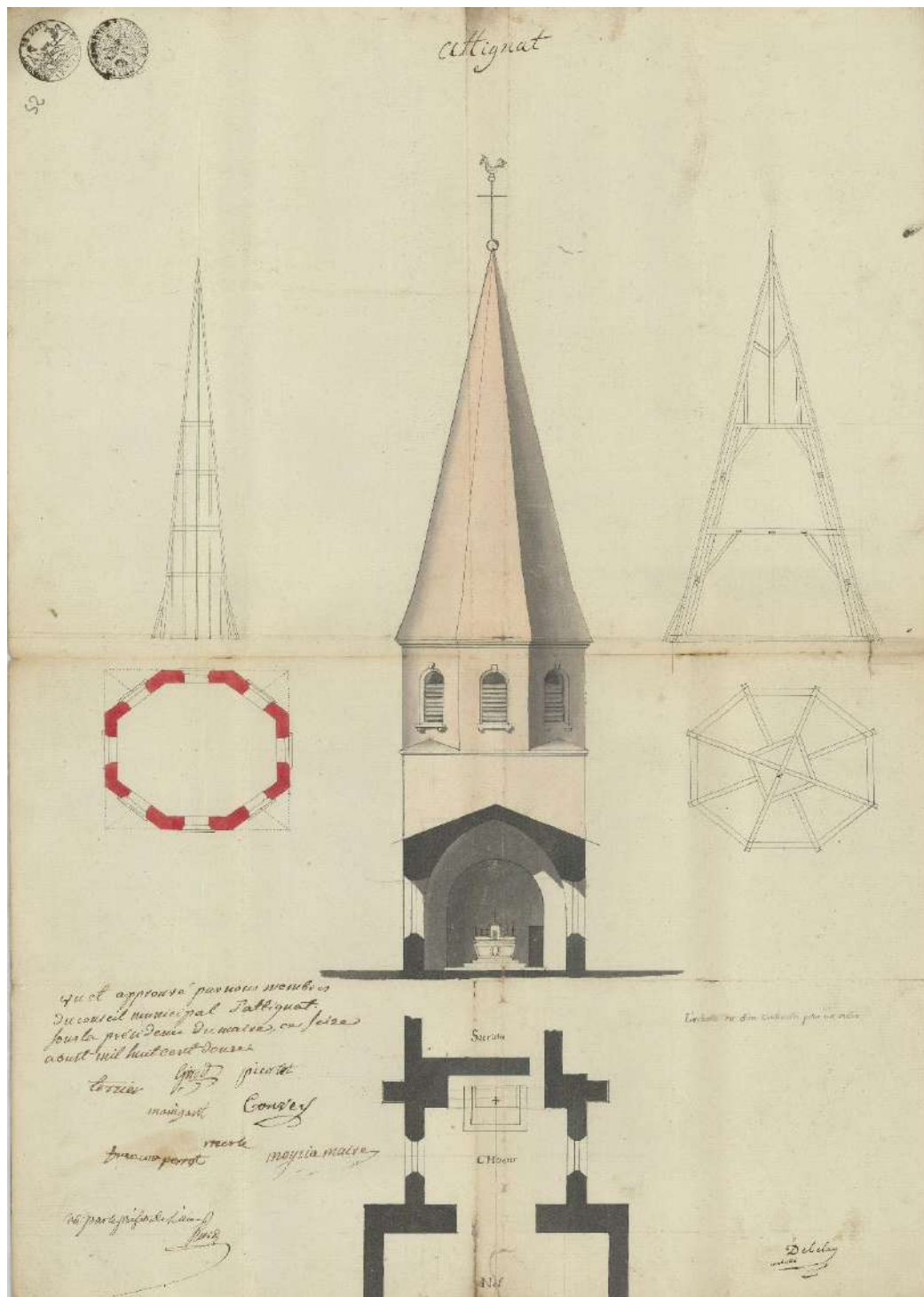
Figure 9 - Plan pour la reconstruction du clocher, mise en place d'une cloche et agrandissement de l'église, Fi 6 (1812).
