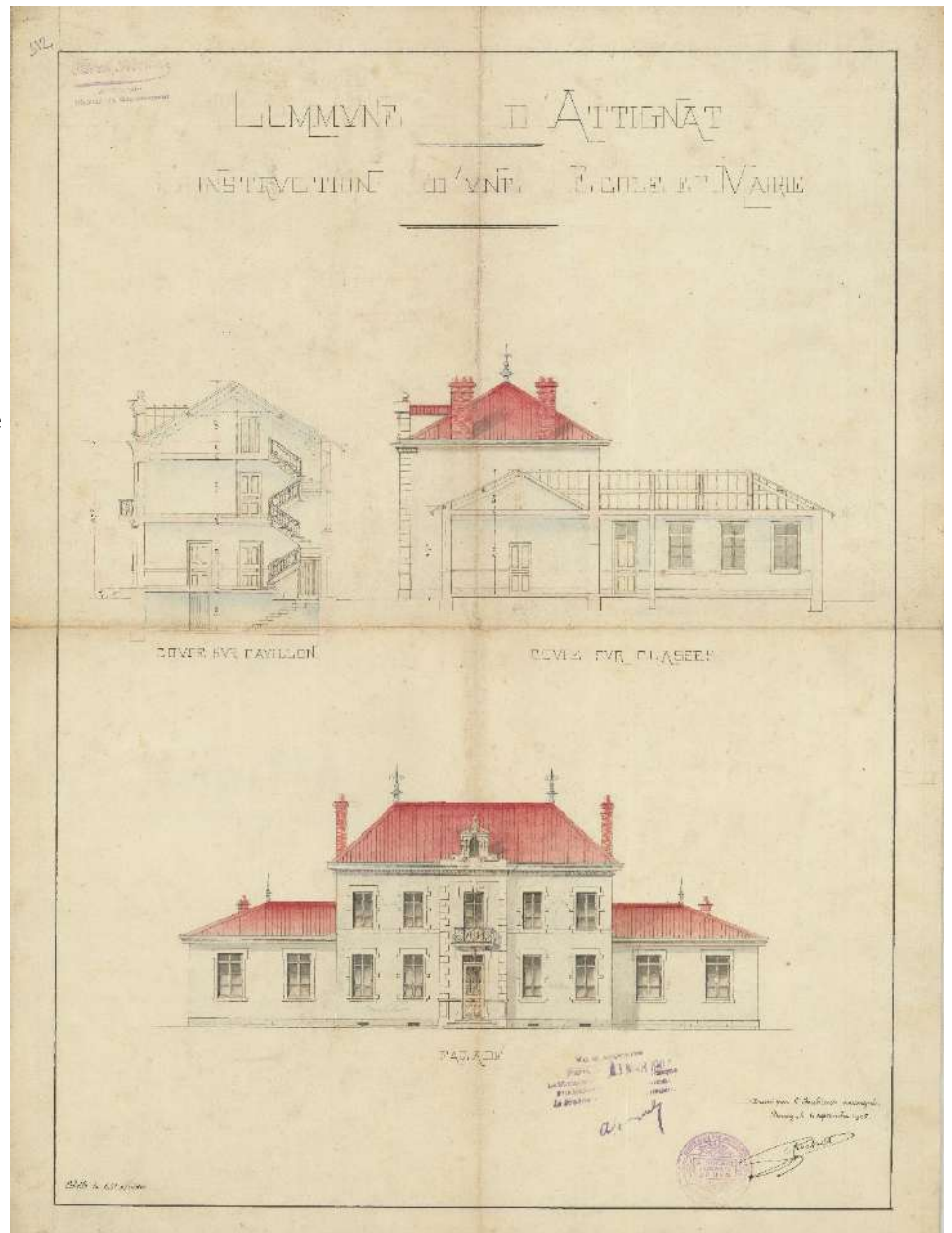
Figure 7 – Plan pour la construction d'une maison d'école (2 nd bâtiment), Fi3 (1905).
