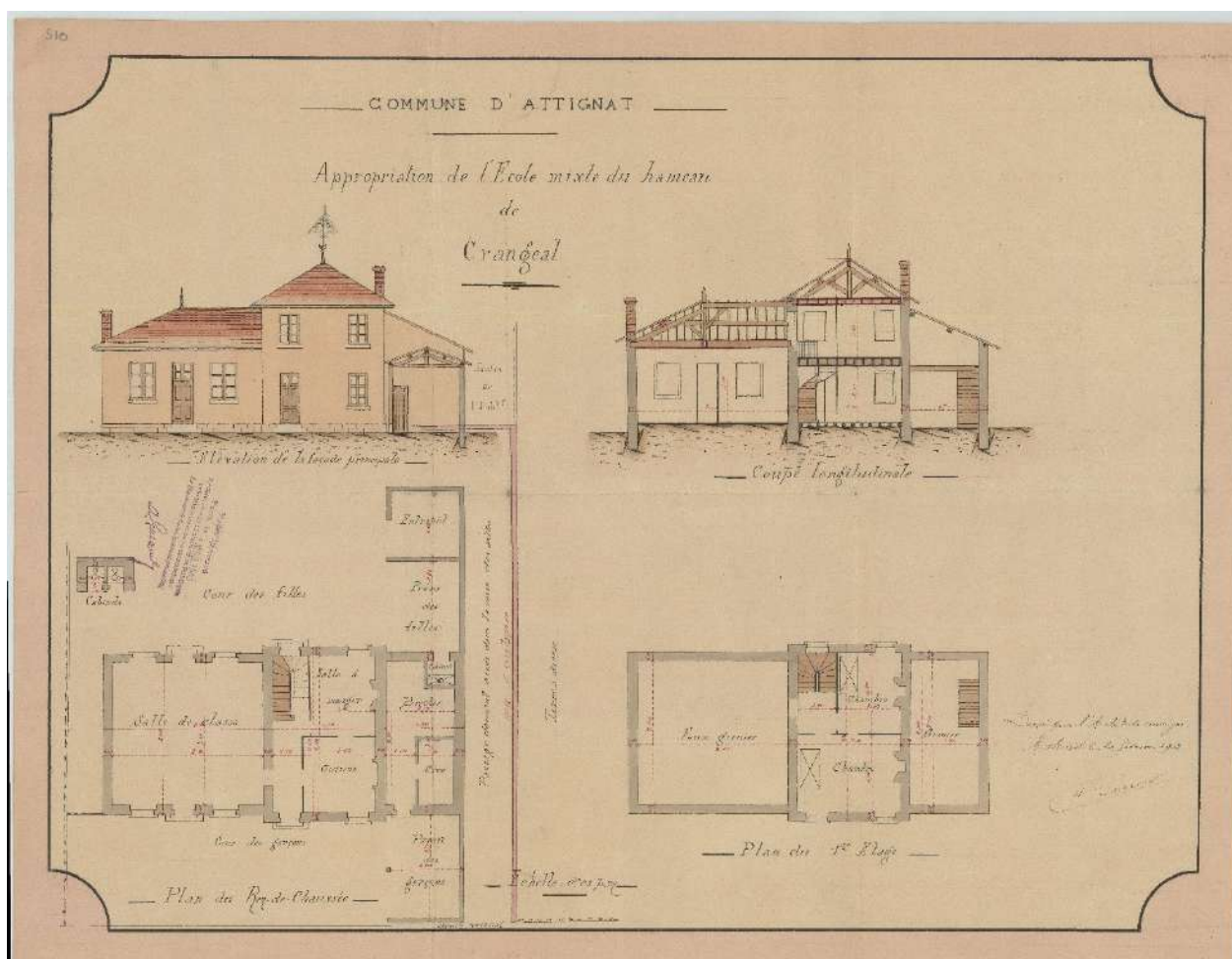
Figure 10 – Plan de l'école de Crangeat pour des travaux d'appropriation de l'école des garçons du bourg et de l'école mixte de Crangeat, Fi7 (1902).
