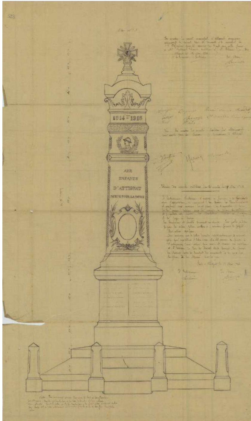
Figure 8 - Plan pour la construction du monument aux morts, Fi4 (1922).
