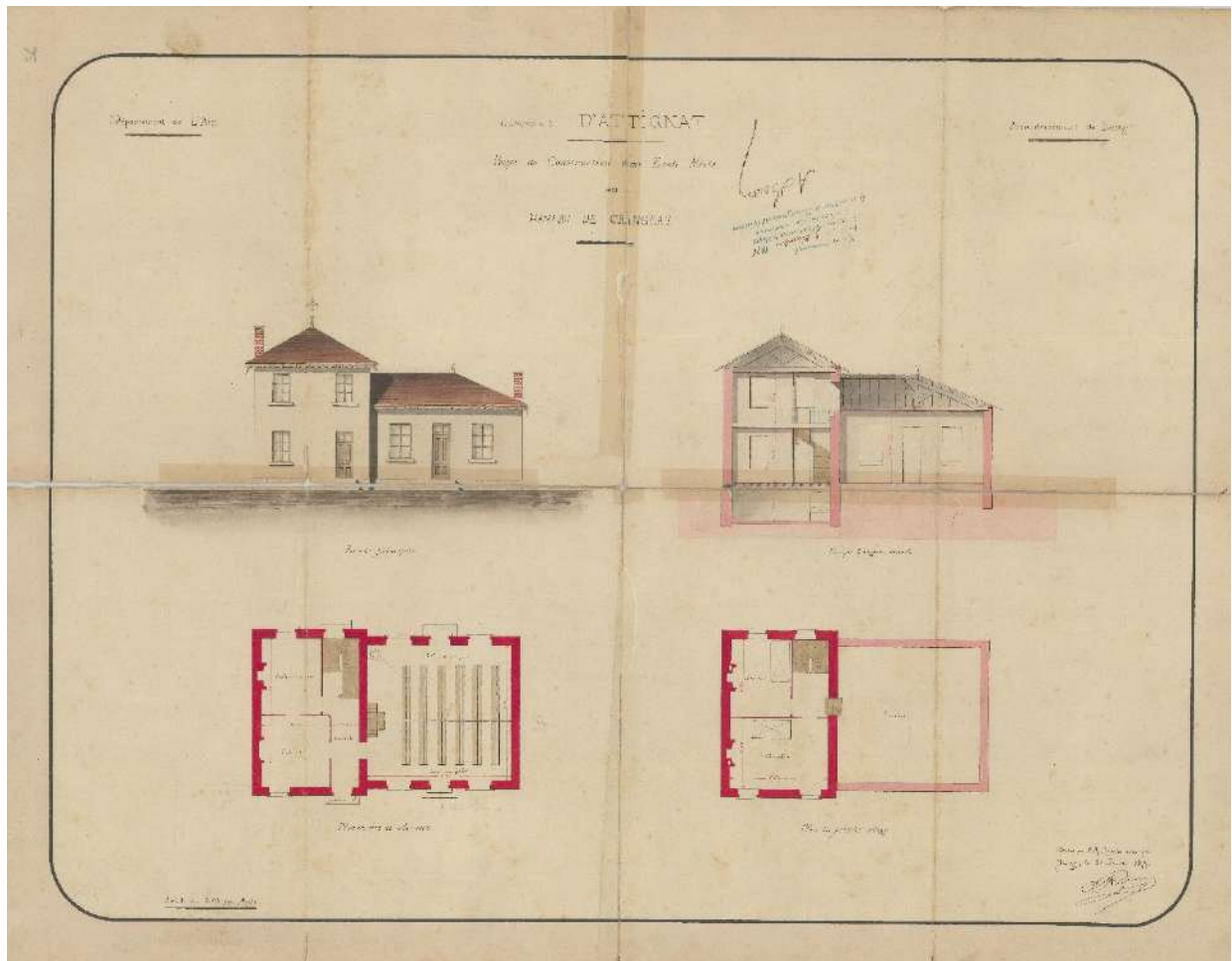
Figure 11 - Plan pour la construction d'une école mixte au hameau de Crangeat, Fi9 (1877).
