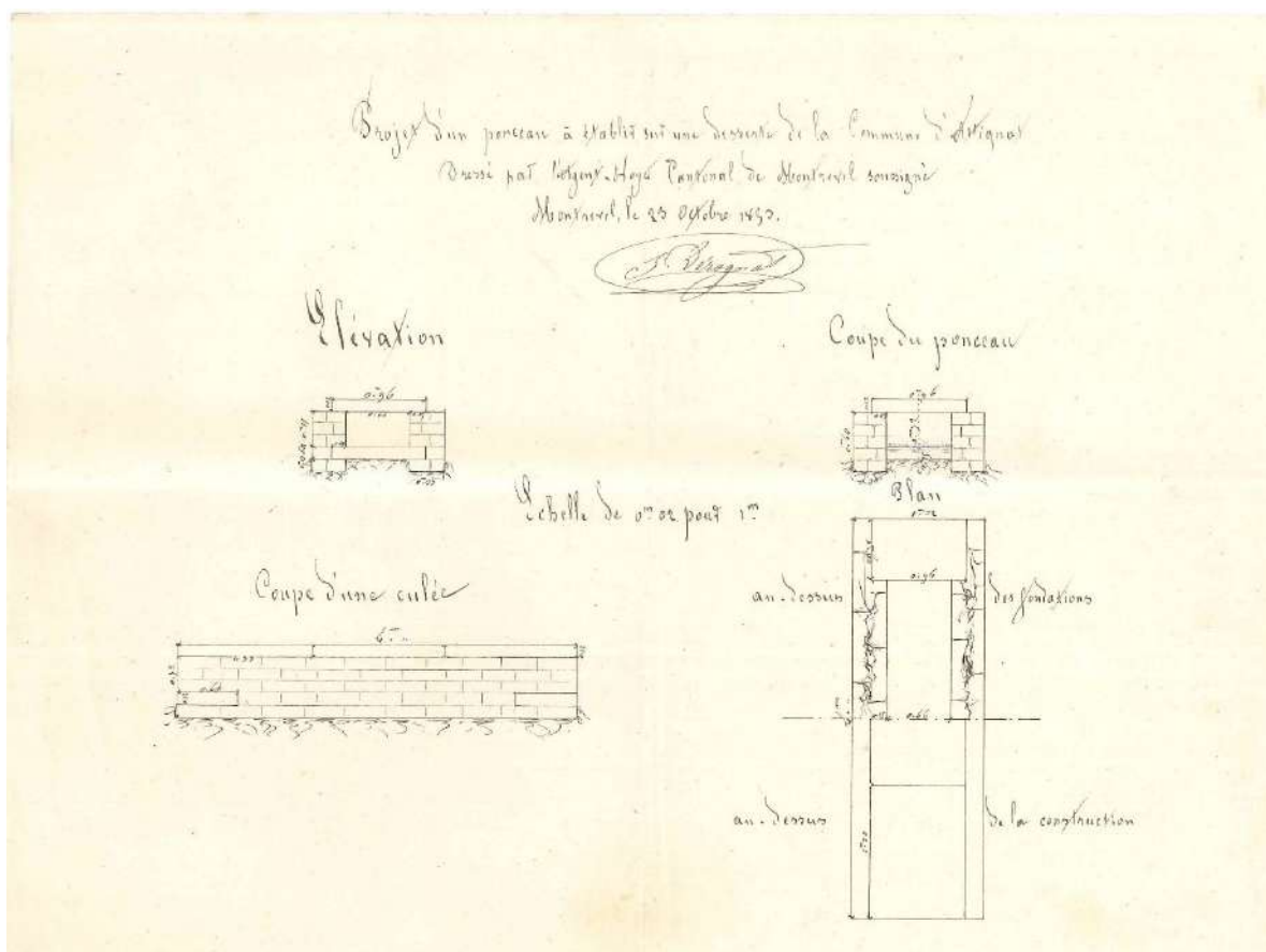
Figure 5 – Plan pour la construction d'un ponceau en pierre, O7 (1853).
