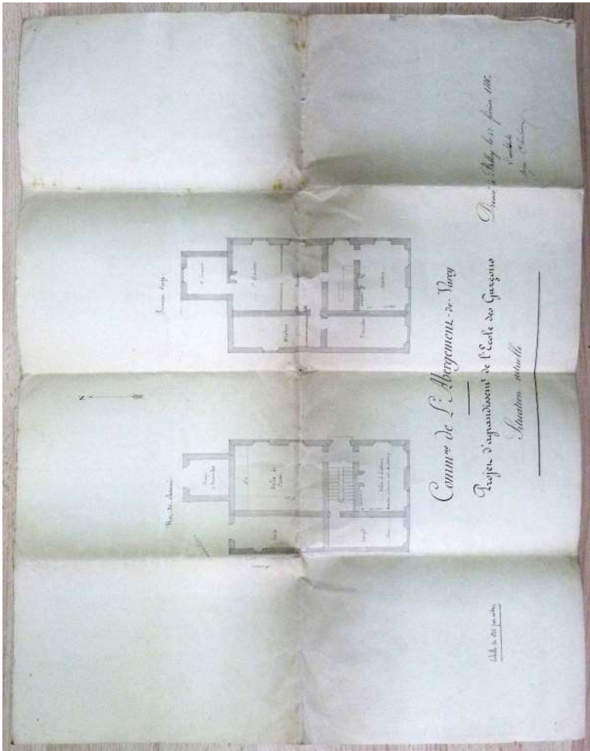
Figure 13 - Plan du projet d'agrandissement de l'école de garçons, 1M1 (1886)
