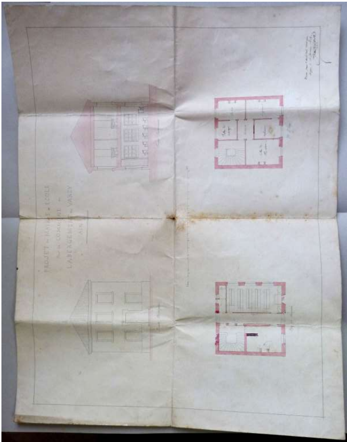
Figure 11 - Plan du projet de construction de la mairie et école, 1M1 (1862)
