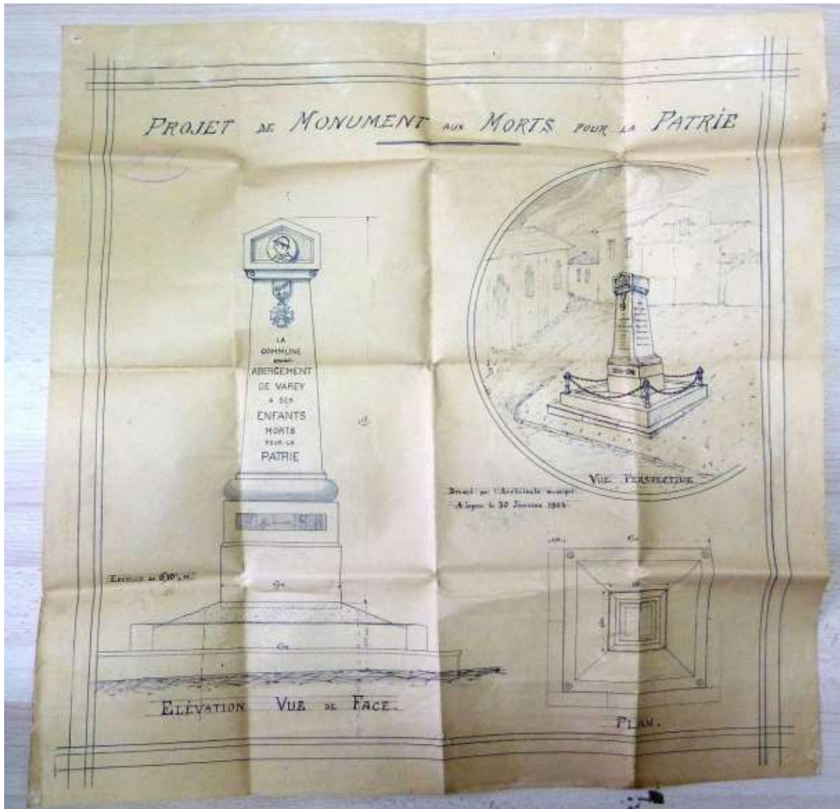
Figure 14 - Plan du projet de monument aux morts, 1M3 (1923)
